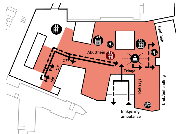
Figur 6.18 Slagsløyfe.
