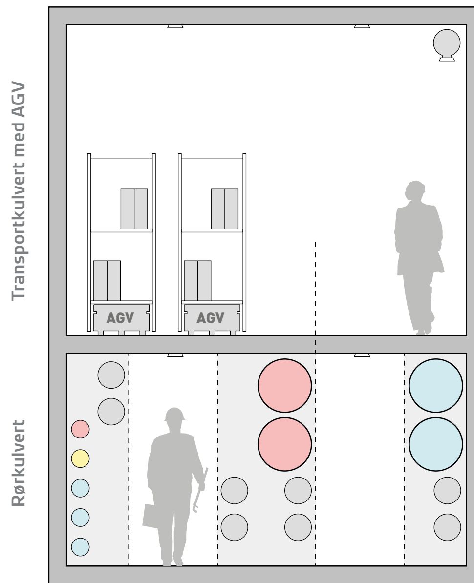
Figur 6.62 Ny transport og teknikkulvert.
