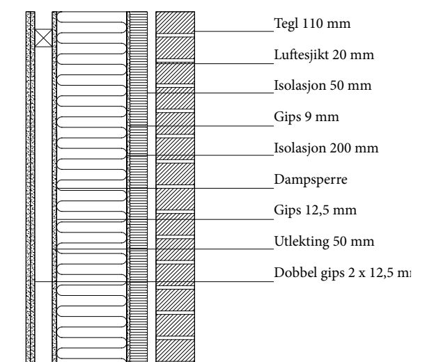
Figur 8.8 Fasadedetalj snitt yttervegg med ekstra lydkrav.
