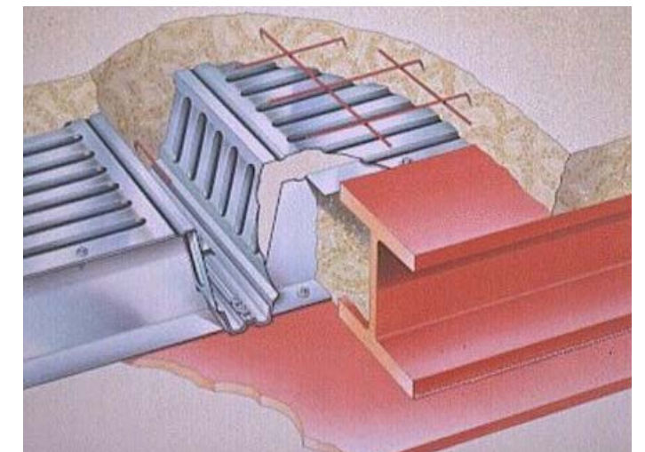
Figur 8.4 Dekker.
