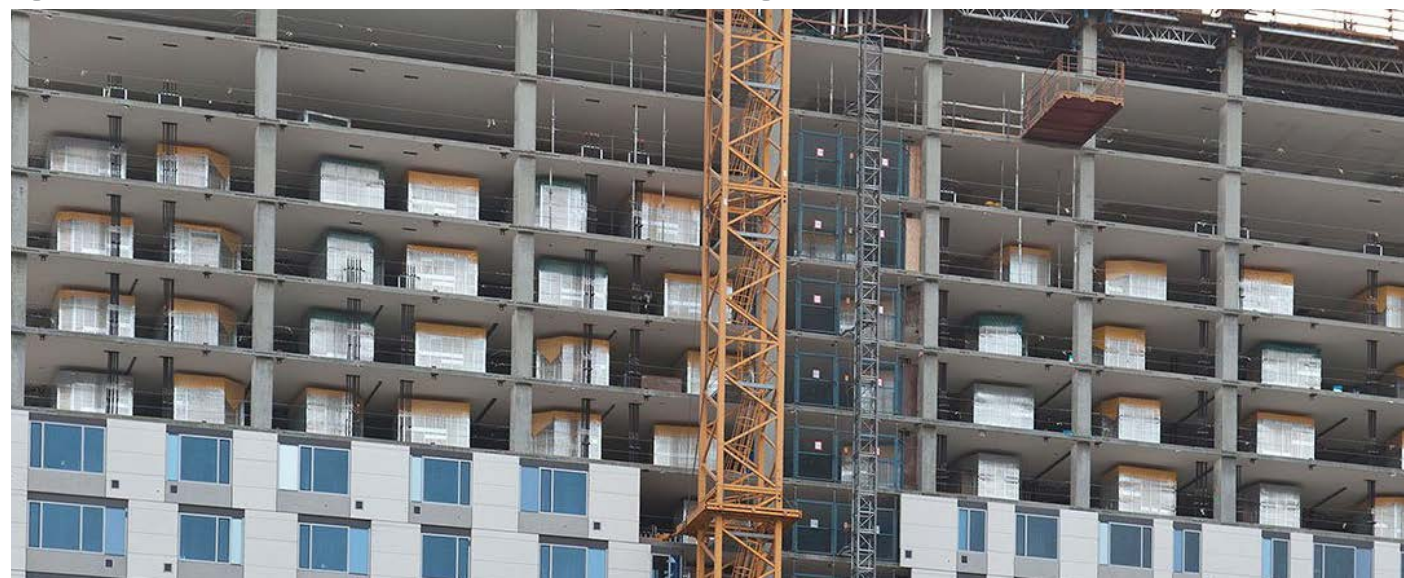
Figur 8.13 Eksempel høybygg med prefabrikkerte elementer.
