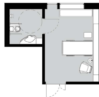
Figur 6.13 Plan rom med mellomliggende bad.
