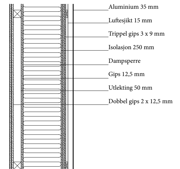
Figur 8.7 Fasadedetalj snitt yttervegg.
