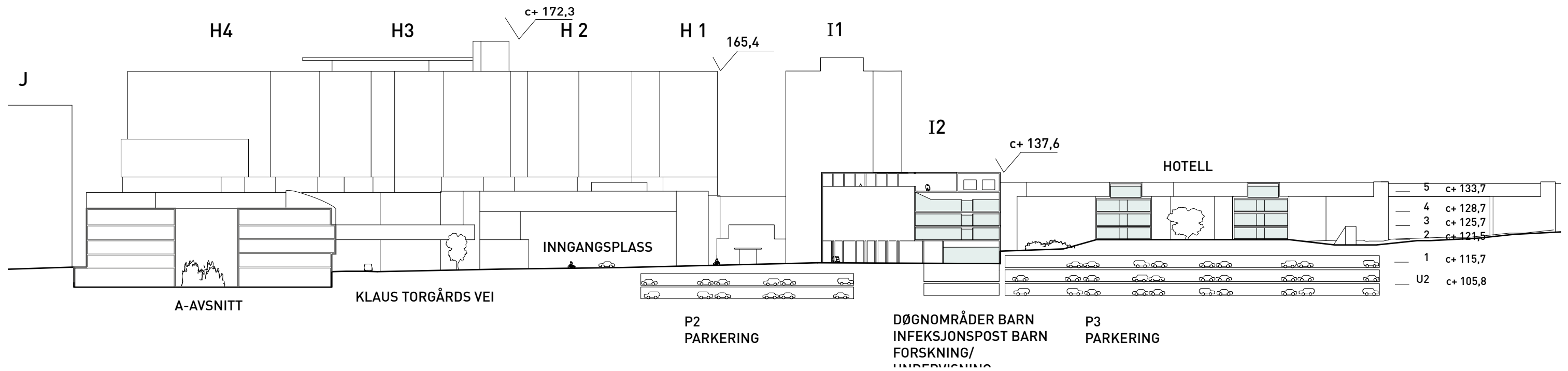
SNITT BB 1:1000
