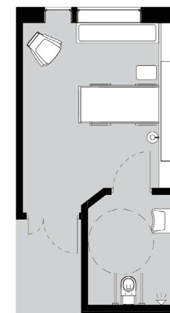
Figur 6.14 Plan rom med bad mot korridor.
