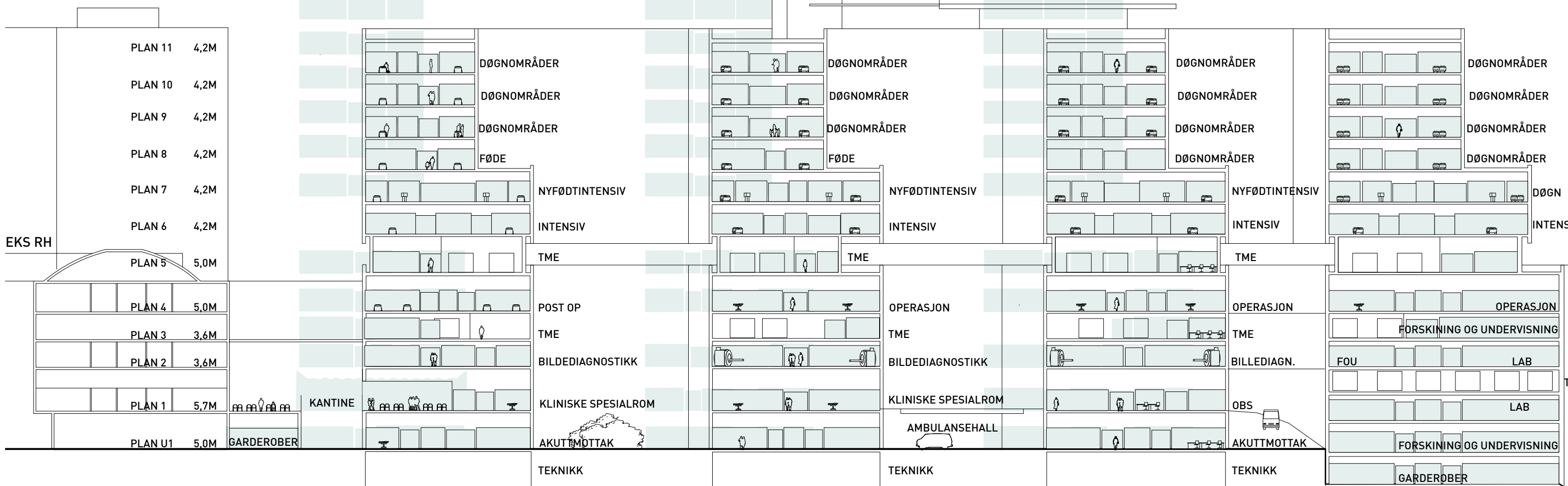
SNITT AA 1:500
