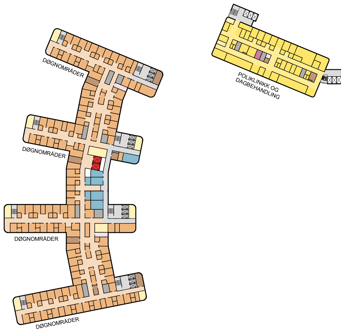
PLAN 11 1:1000
