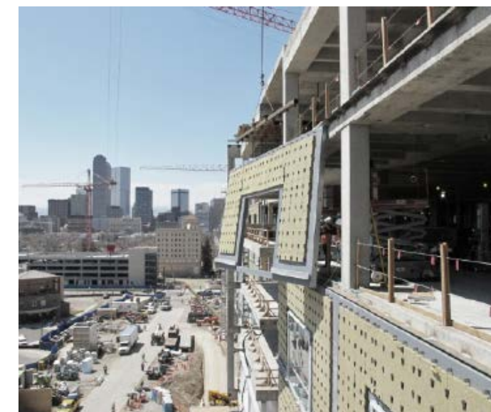
Figur 8.12 Eksempel prefabrikkerte fasadelementer.
