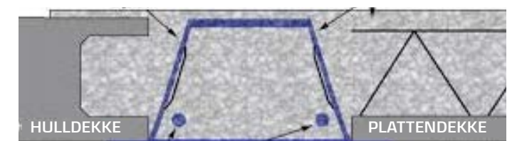
Figur 8.5 Konstruksjon.
