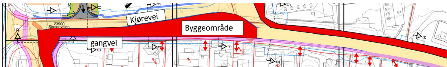
Situasjonsplan fase 1.5 etter omlagt kjørevei søndre del.
